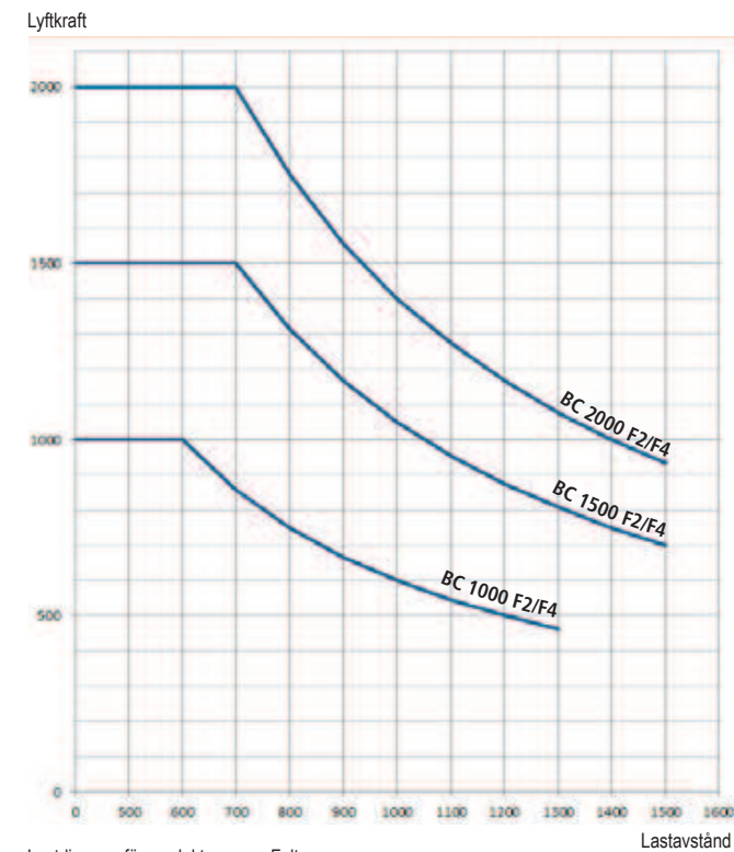
Lastdiagram för produktgruppen Falt
